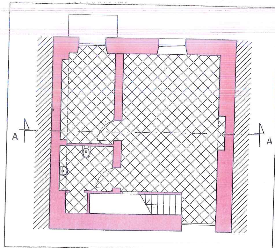
PIANTA PIANO TERRA quota 0,00 RAPP. 1:100
