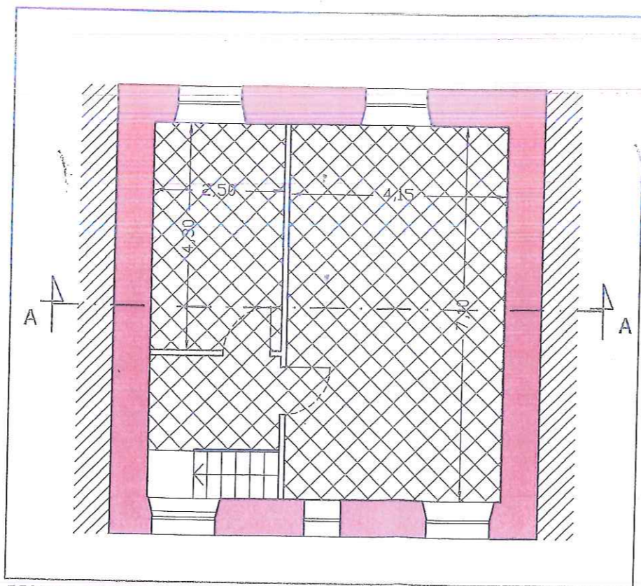
PIANTA PIANO PRIMO quota 3,20 RAPP. 1:100
