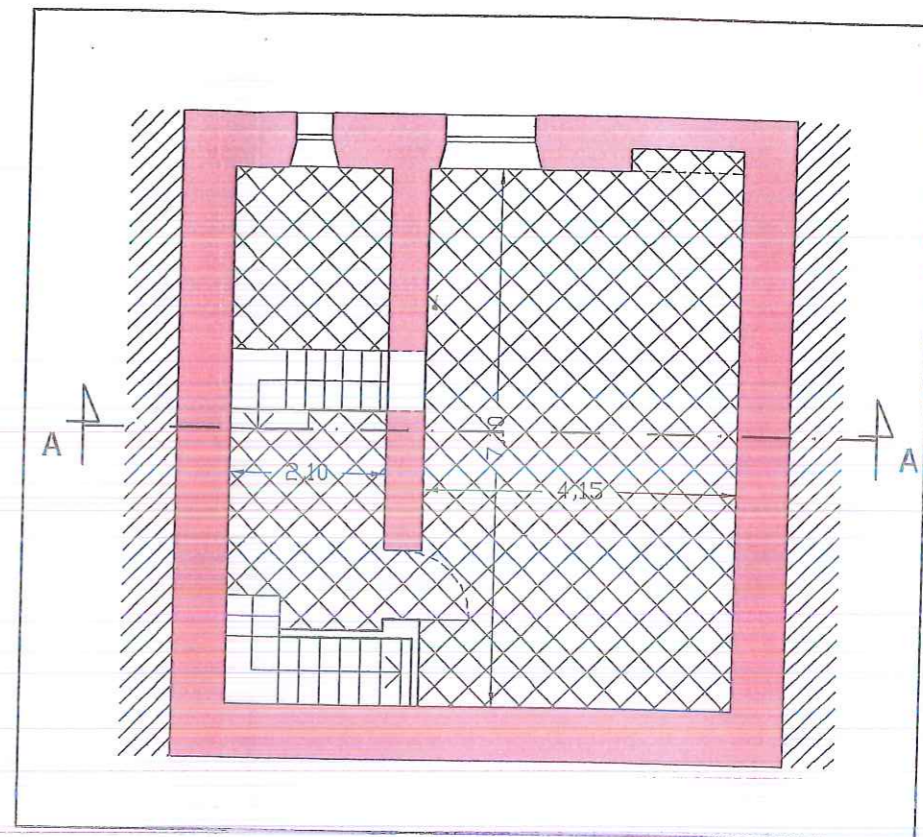
PIANTA PIANO SEMINTERRATO quota - 3,20 RAPP. 1:100
