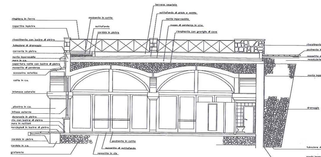
SEZIONE A-A
