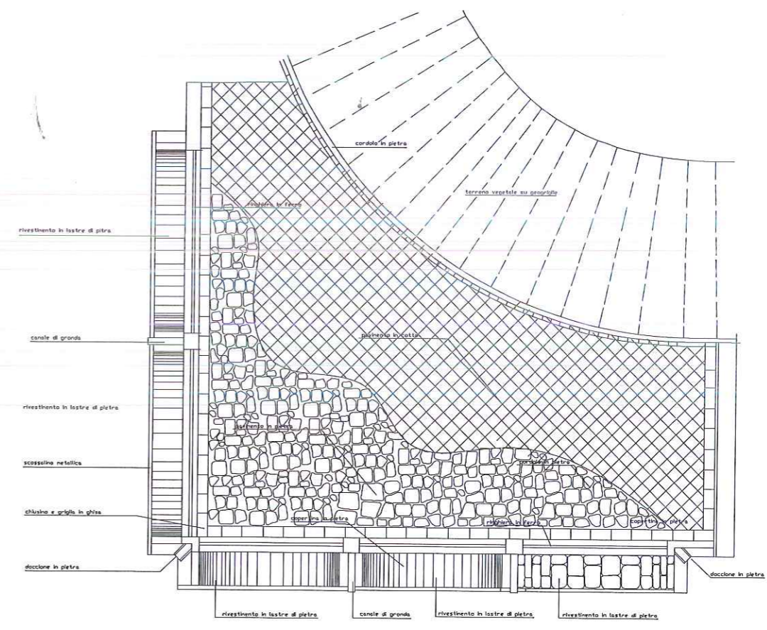
PIANTA COPERTURA
