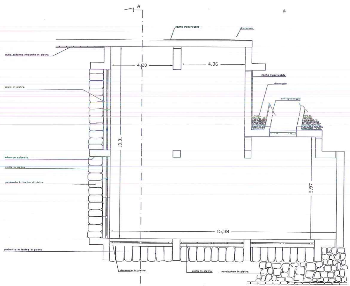
PIANTA scala 1:50
